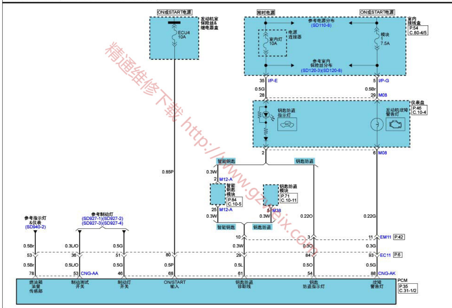
发动机控制系统(G4NA : NU 2.0L MPI A/T )(7)
